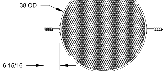
IAFS-30 LID
